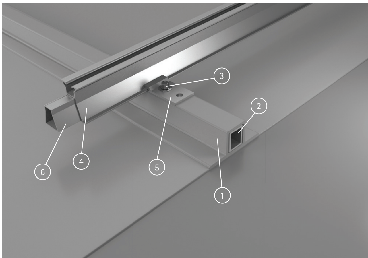
Componentes del sistema RENOLIT ALKORPLAN Solar
