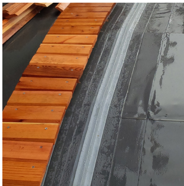
Listones de madera fijados a los perfiles RENOLIT ALKORPLAN Solar .
